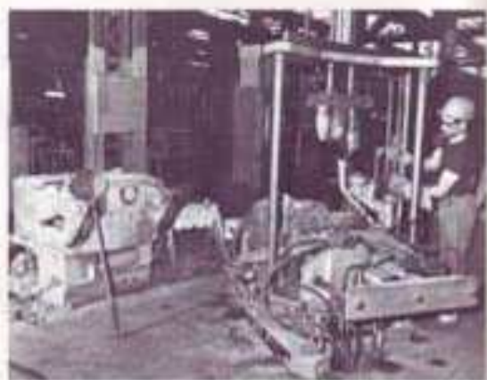
L'atelier d'assemblage et de mise en place des noyaux sur la chaîne des moules du carter-moteur. La fonte liquide s'insinuera dans les espaces laissés libres par les noyaux de sable aggloméré.
